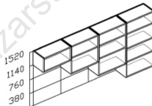
NASTAVNI ELEMENTI BREZ VRAT 800 mm x višina x 380 mm
