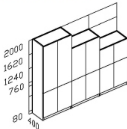
KOMBINIRANI ELEMENTI Z VRATI 800 mm x višina x 400 mm
